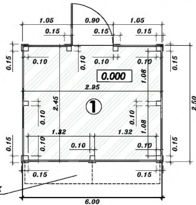
План на відм. 0.000 М 1:50
